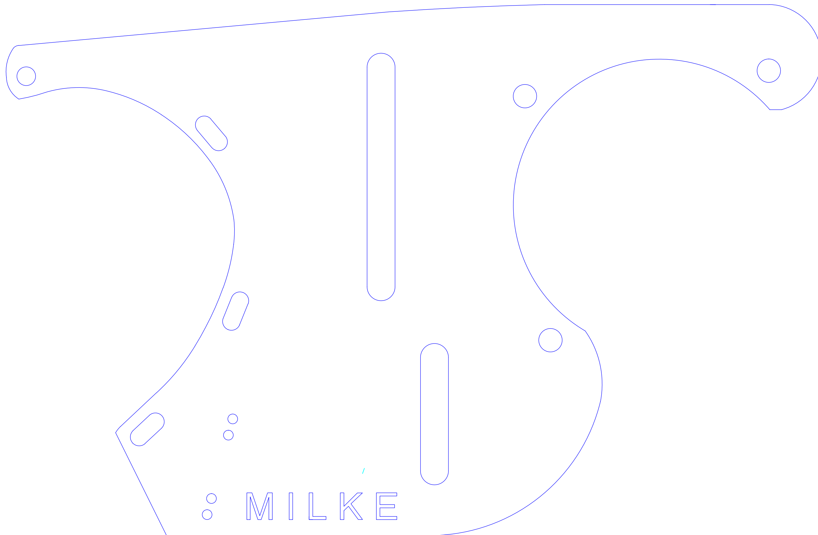
Chapa compressor - aço chapa preta espessura 6,0 mm - Escala 1:1 mm
